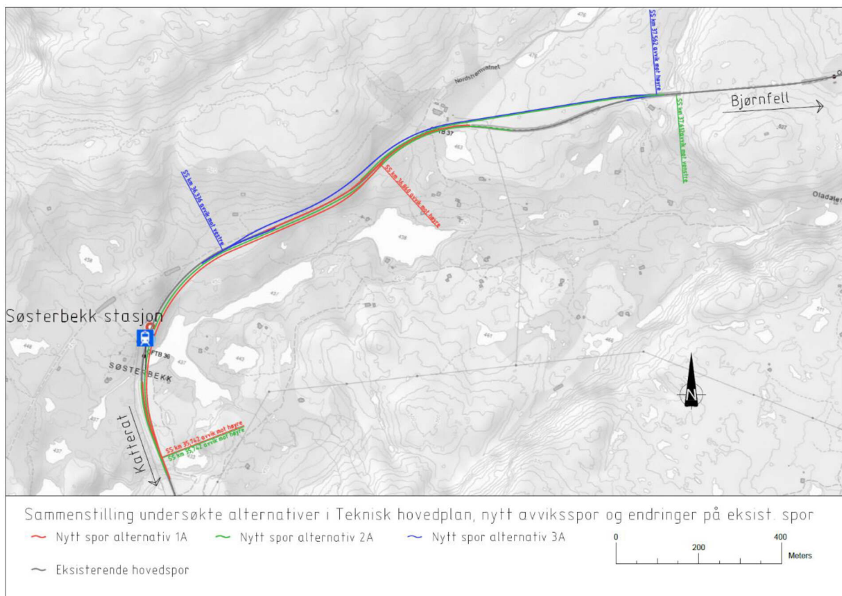
Figur 7 Viser alternativ 1A, 2A og 3A
