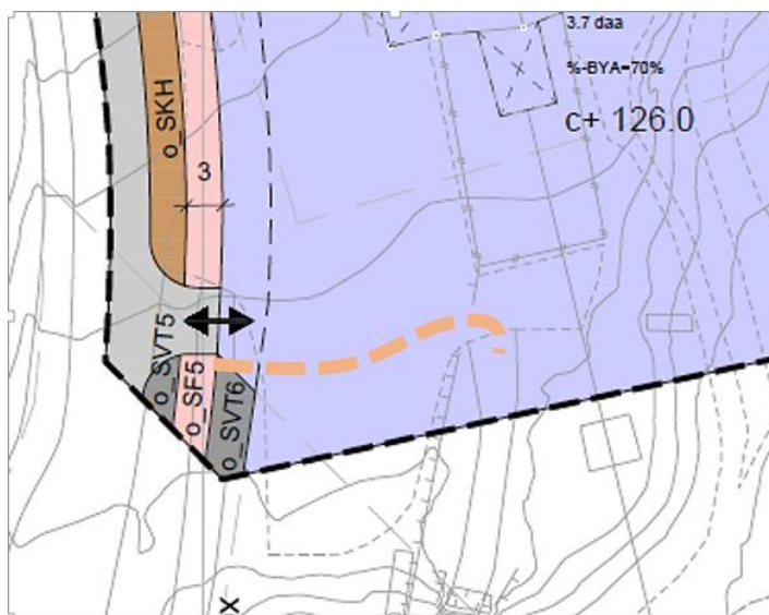
Figur 6-6: Illustrasjon av gangforbindelse mellom Skistuaveien og gangkulvert.
