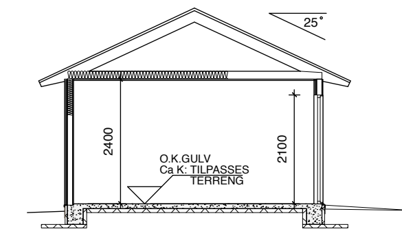
SNITT A-A
