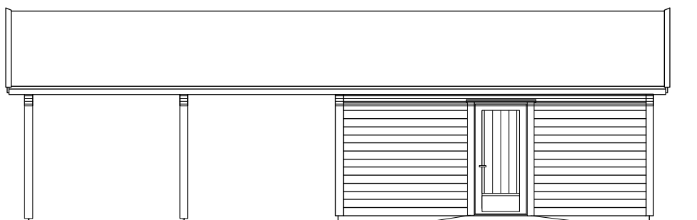
BOD A: FASADE MOT SØR
