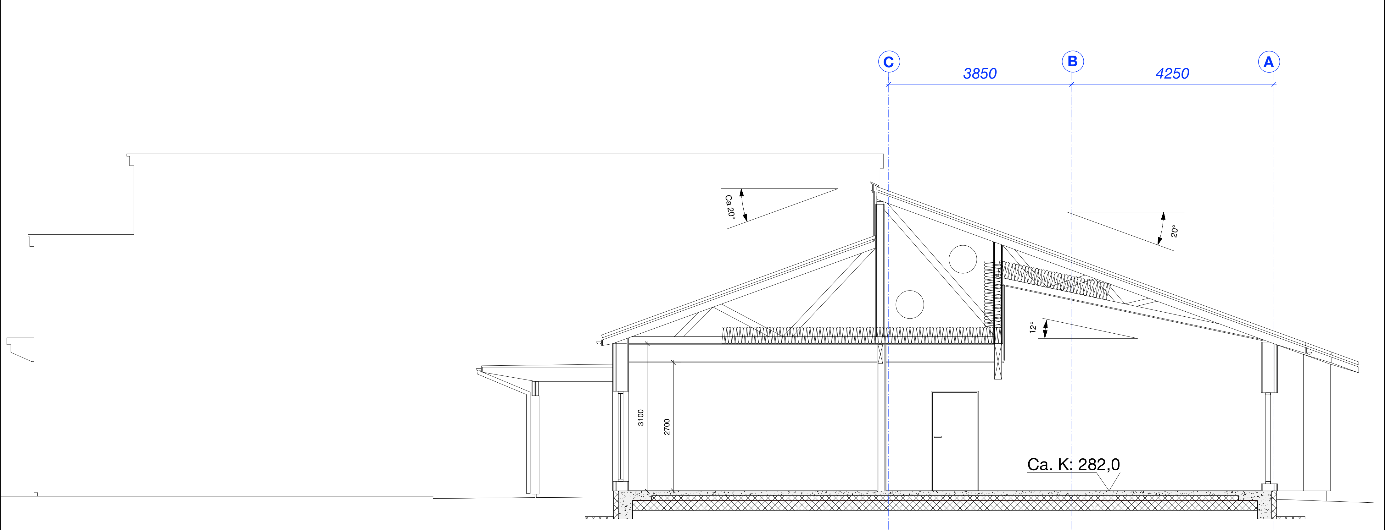
SNITT A-A
