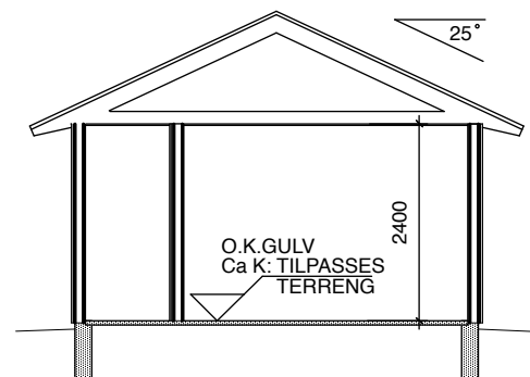
SNITT B-B
