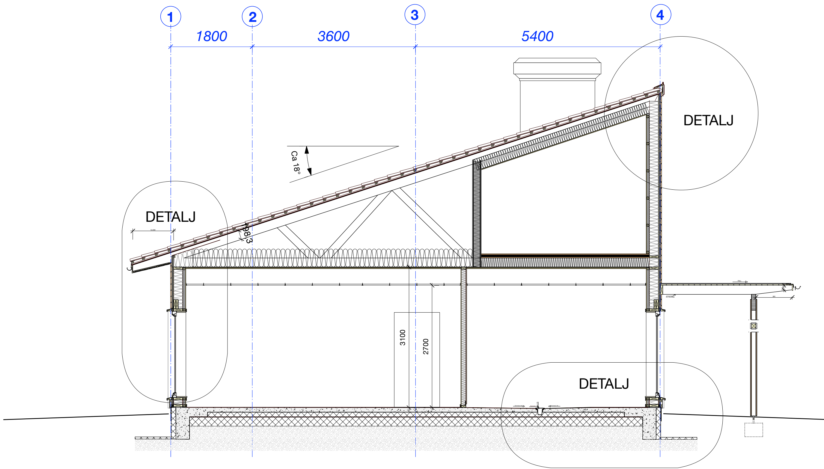
SNITT B-B
