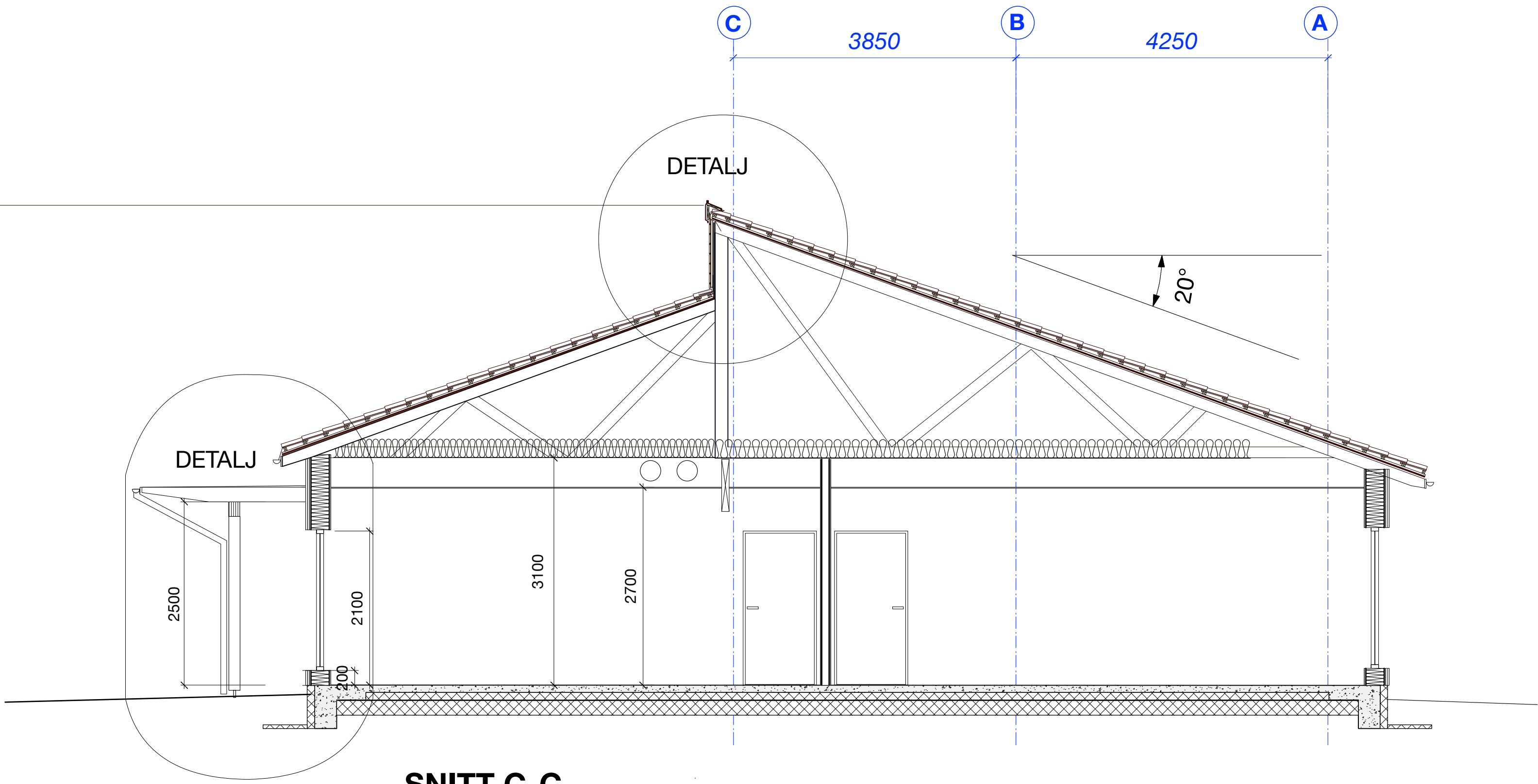
SNITT C-C
