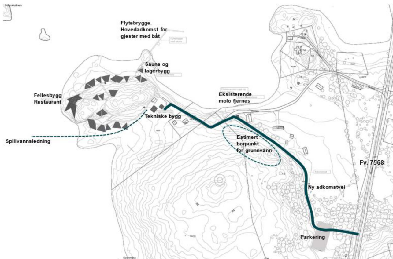
Figur 5. Skisse over planforslaget, underlag fra Snøhetta arkitekter 5.3.2026. Ny bebyggelse med mørkegrå farge.
