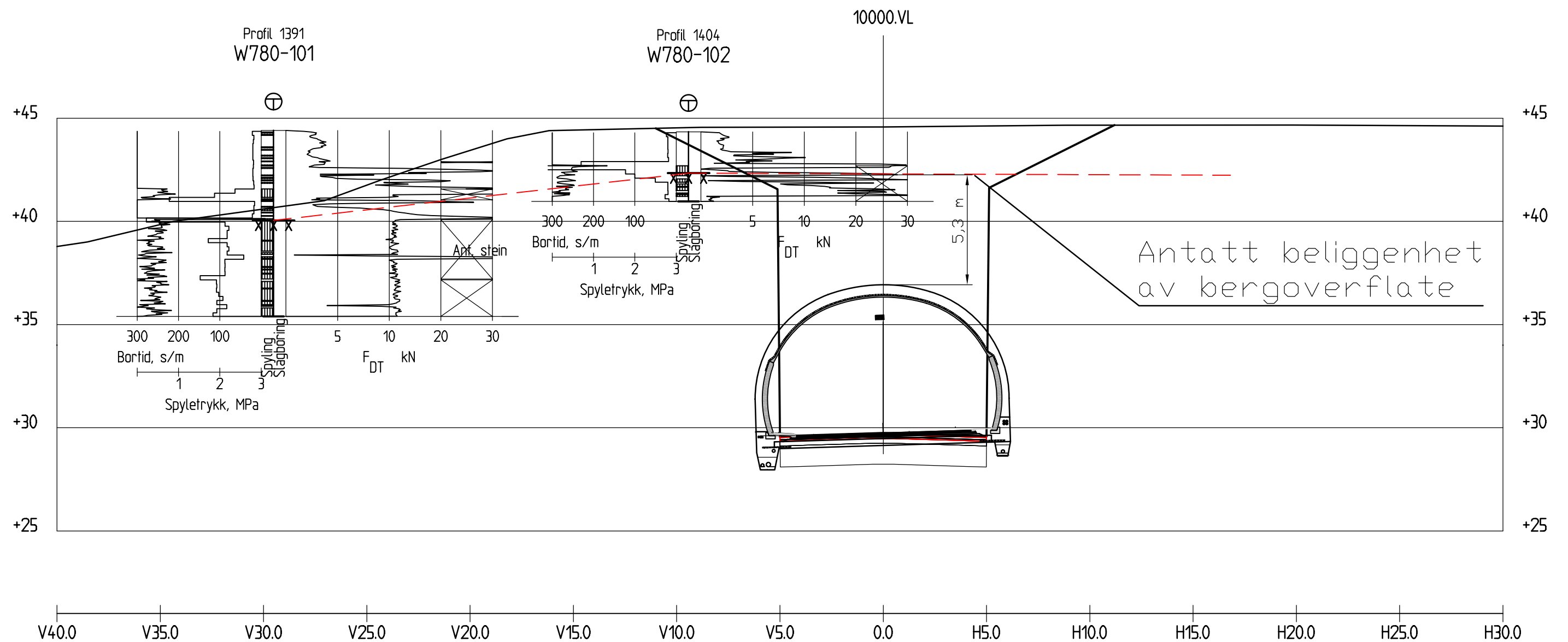
Profil 1400 1 : 200
