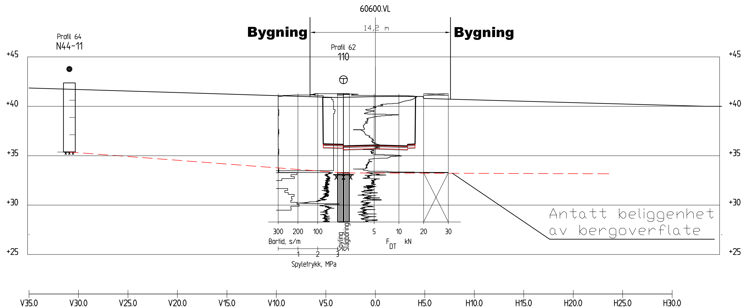
Profil 60 1 : 200
