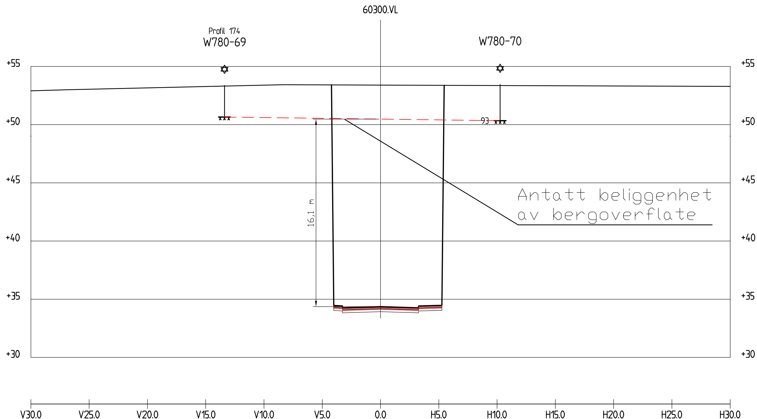
Profil 170 1 : 200
