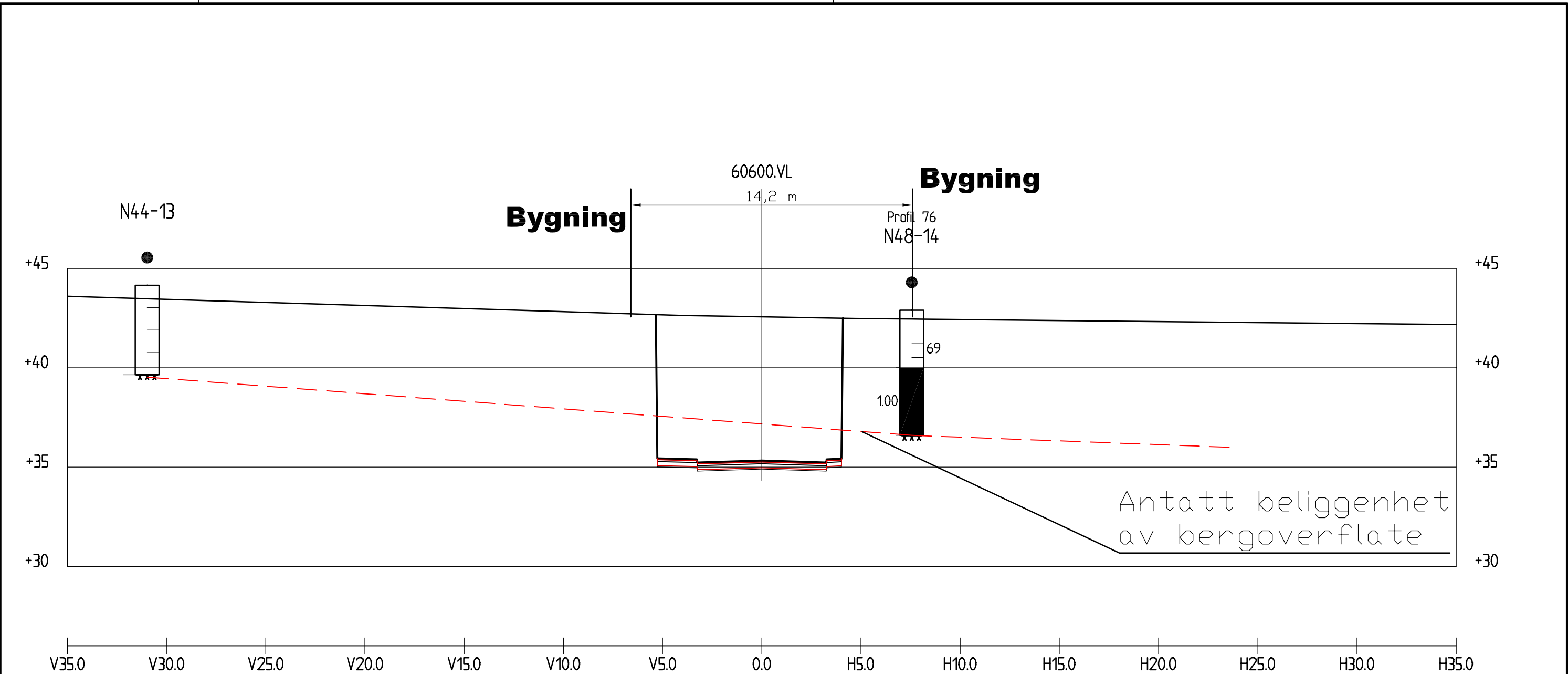
Profil 75 1 : 200
