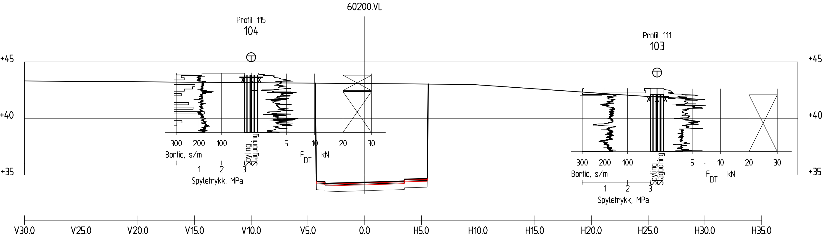
Profil 110 1 : 200
