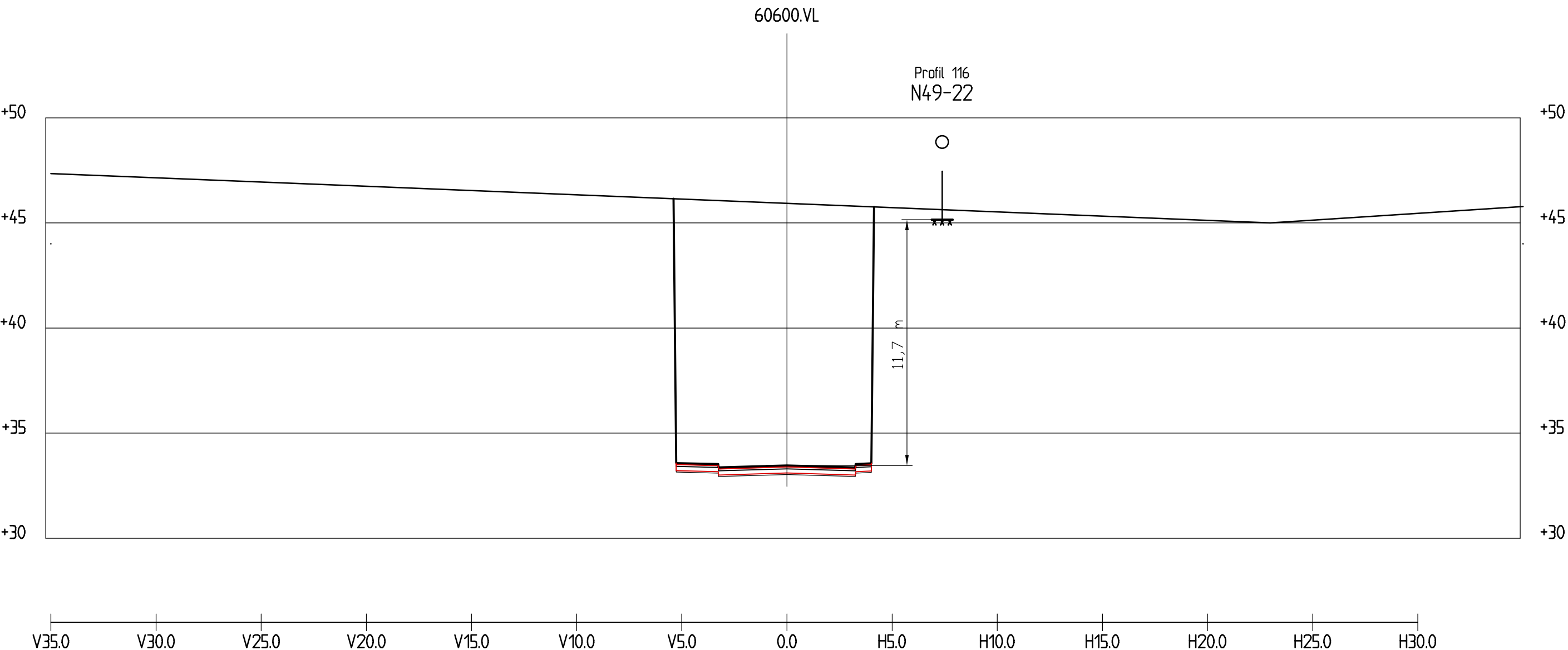
Profil 115 1 : 200
