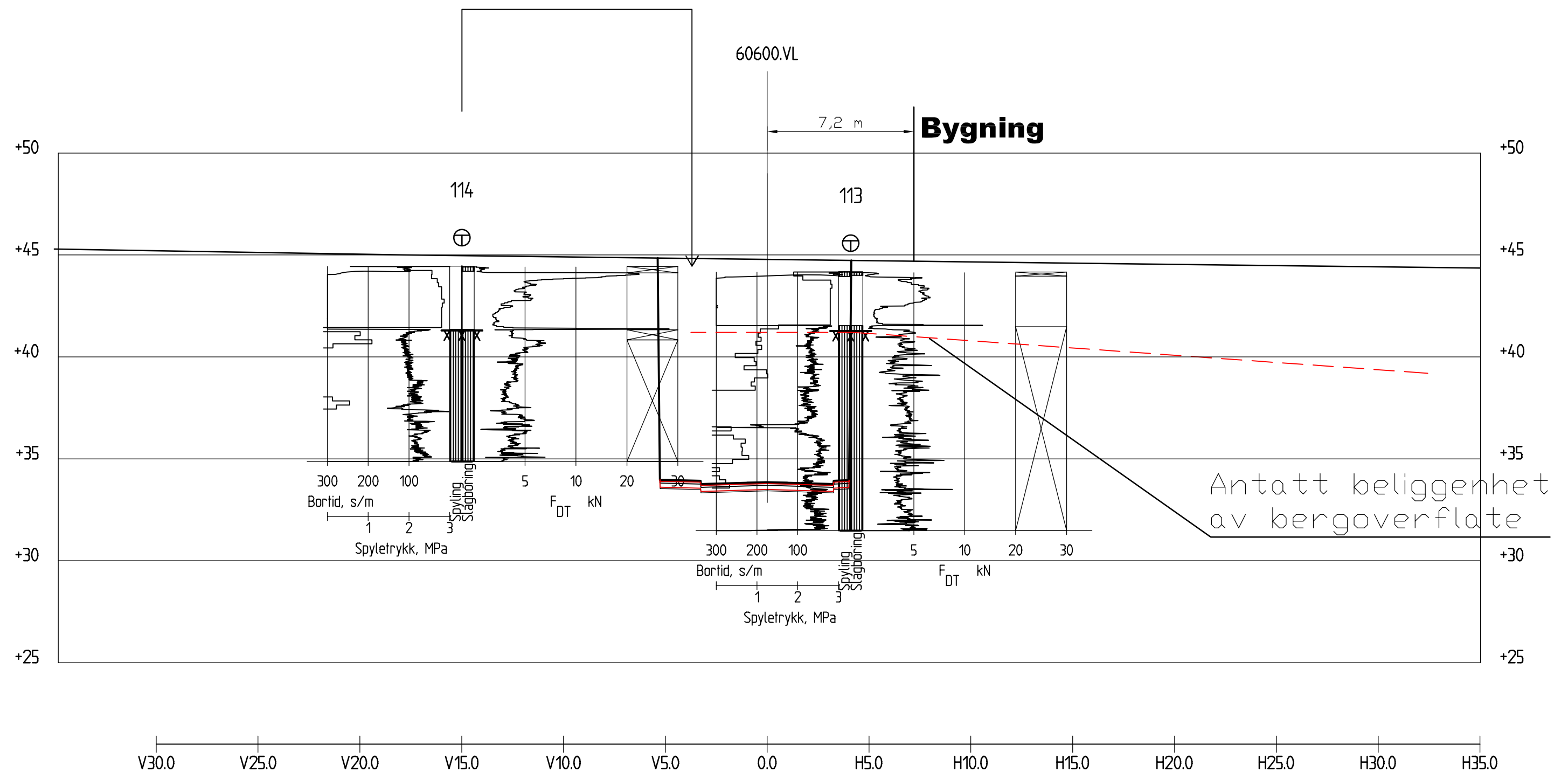
Profil 105 1 : 200
