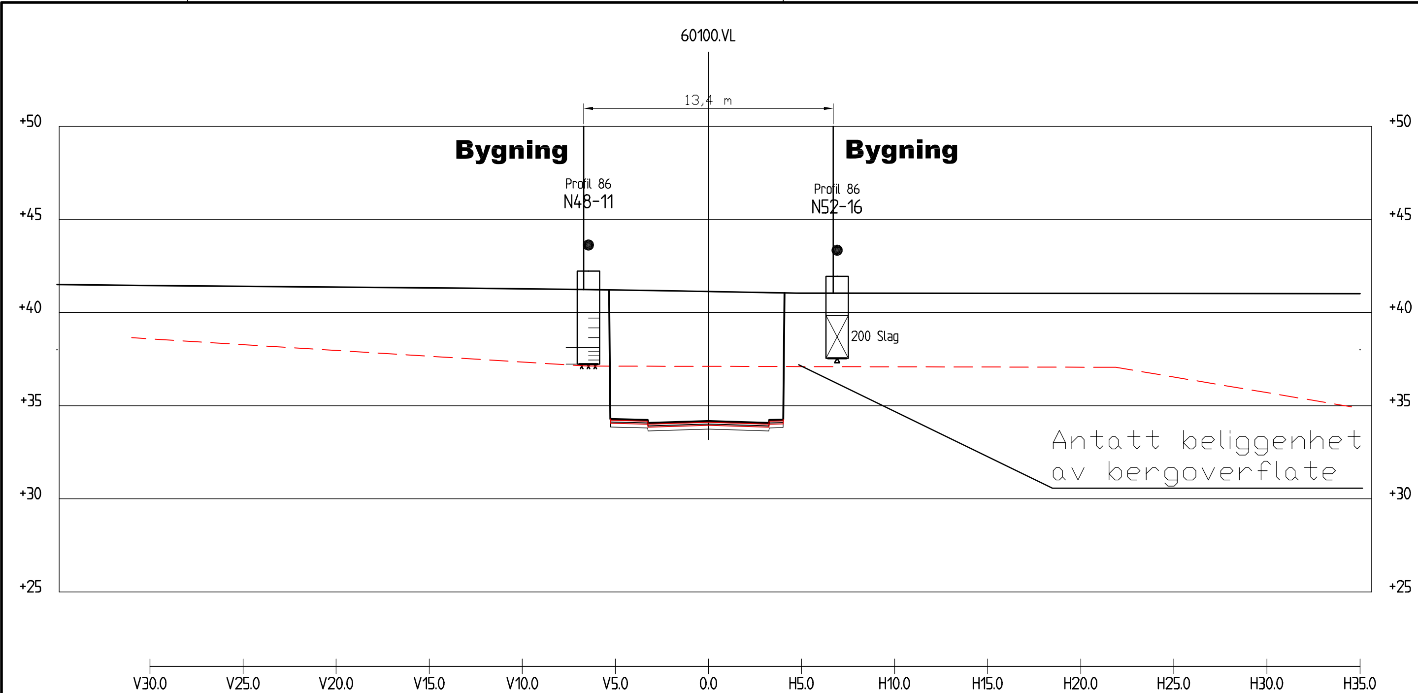
Profil 80 1 : 200
