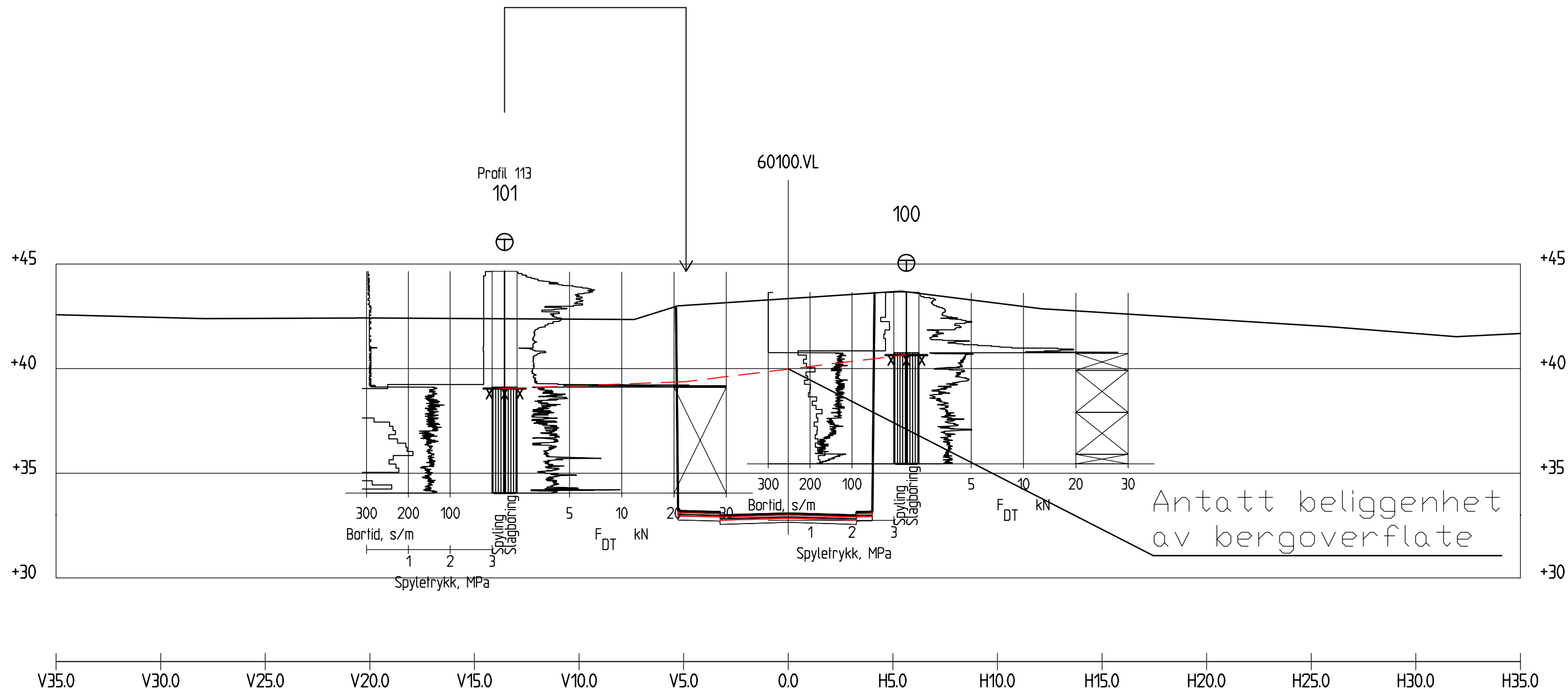
Profil 110 1 : 200
