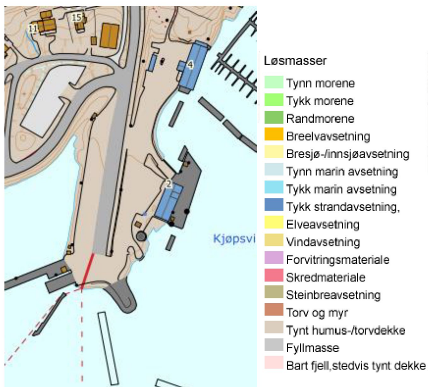
Figur 4: Løsmassekart fra NGU
