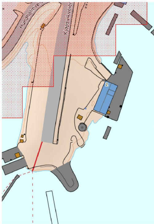
Figur 3: Aktsomhetsområde for snø- og steinskred. Hentet fra DSBs kartinnsynsløsning.
