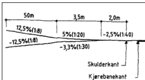
Figur 2: Krav til stigningsforhold på avkjørsel (lengdeprofil)
