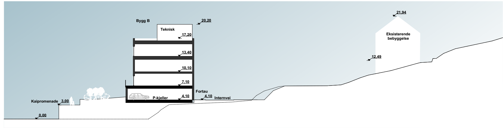
Snitt C
