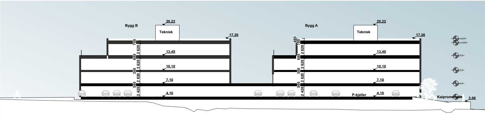
Snitt A
