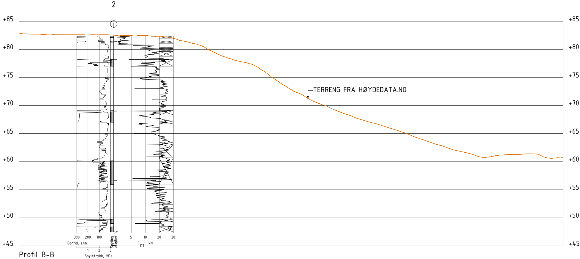
Profil B-B
