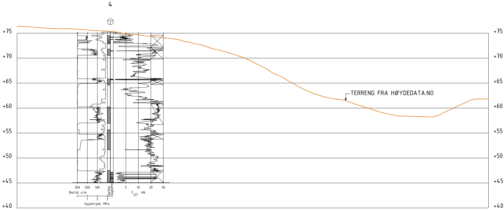
Profil A-A
