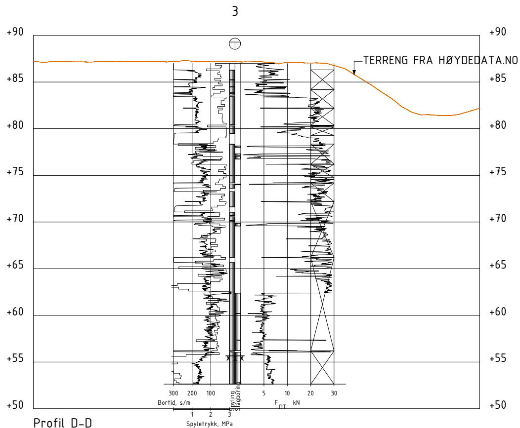
Profil D-D
