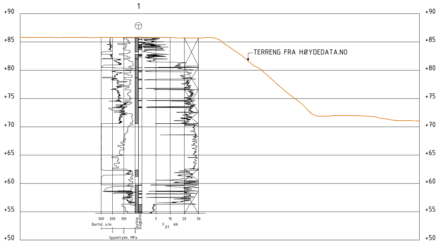
Profil C-C
